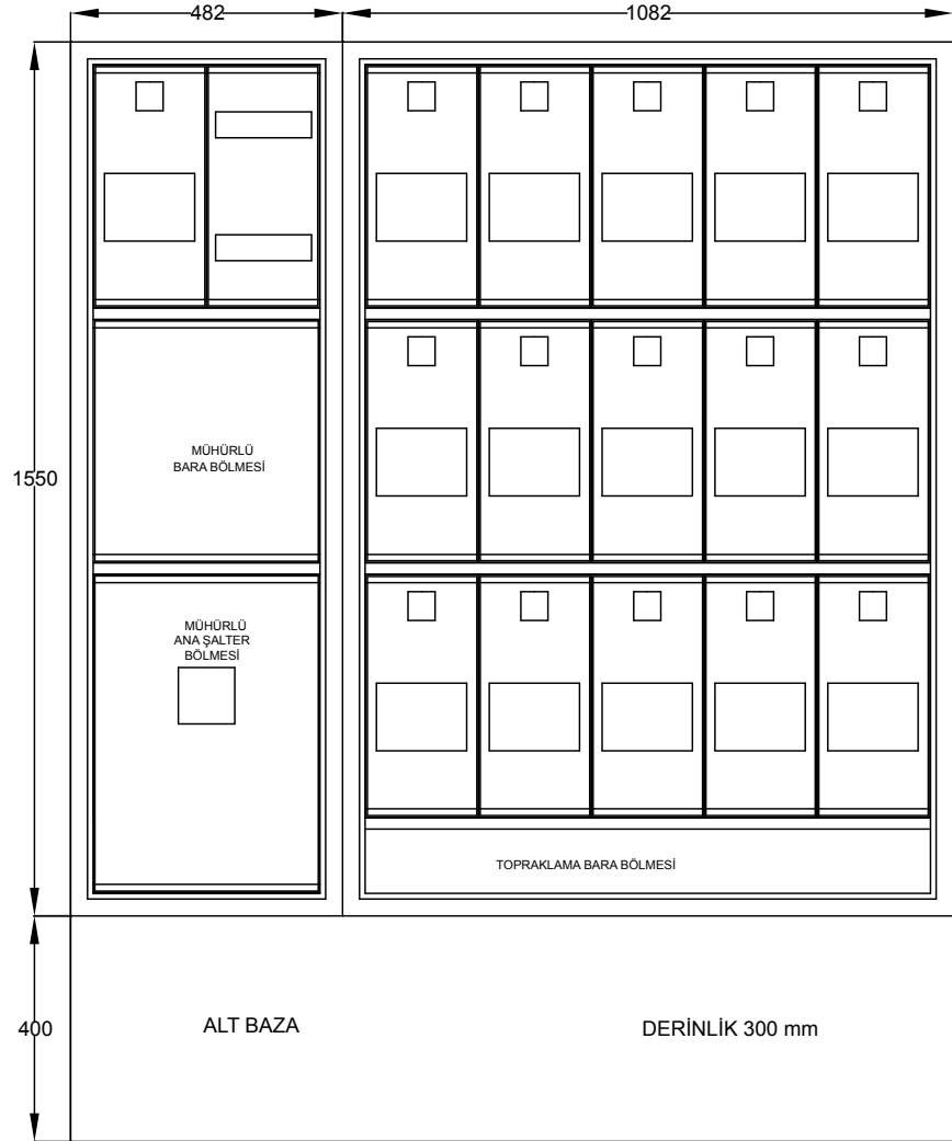
16 TRİFAZE SAYAÇLI DAĞITIM PANOSU
