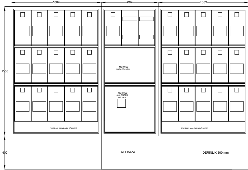
31 TRİFAZE SAYAÇLI DAĞITIM PANOSU
