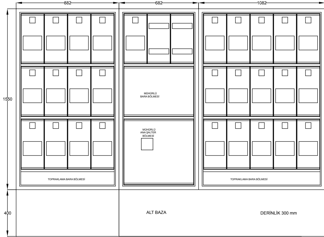
28 TRİFAZE SAYAÇLI DAĞITIM PANOSU
