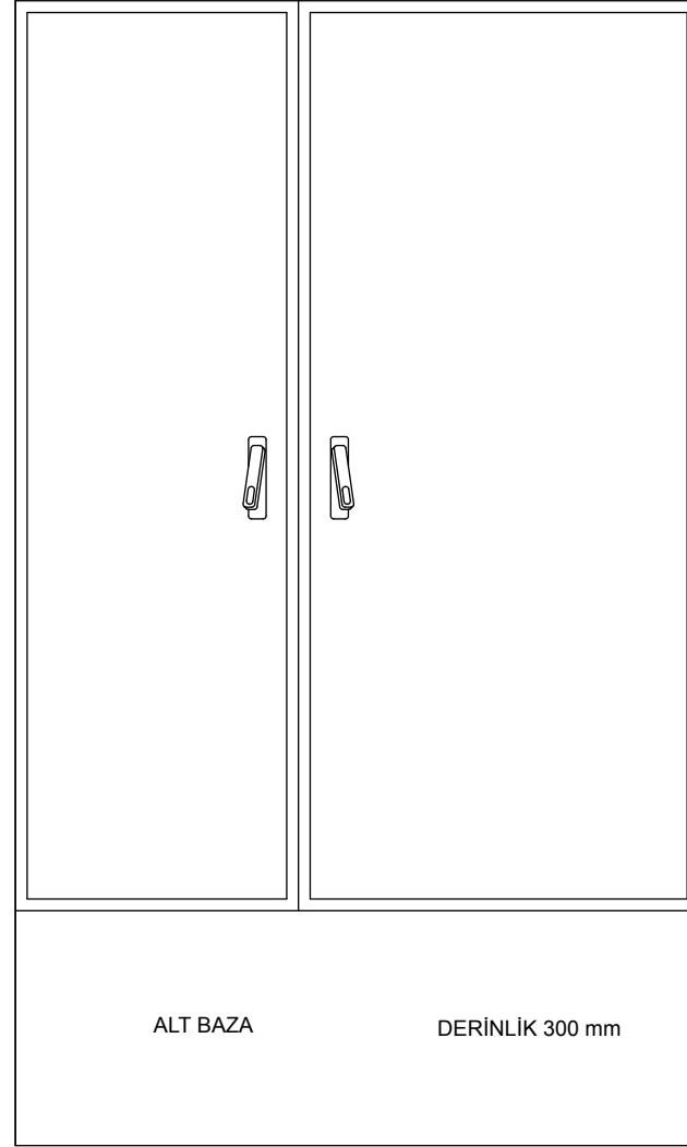
10 TRİFAZE SAYAÇLI DAĞITIM PANOSU
