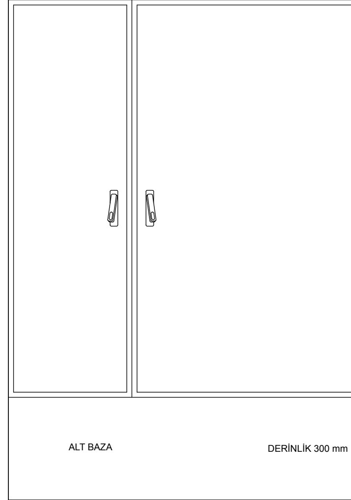
13 TRİFAZE SAYAÇLI DAĞITIM PANOSU
