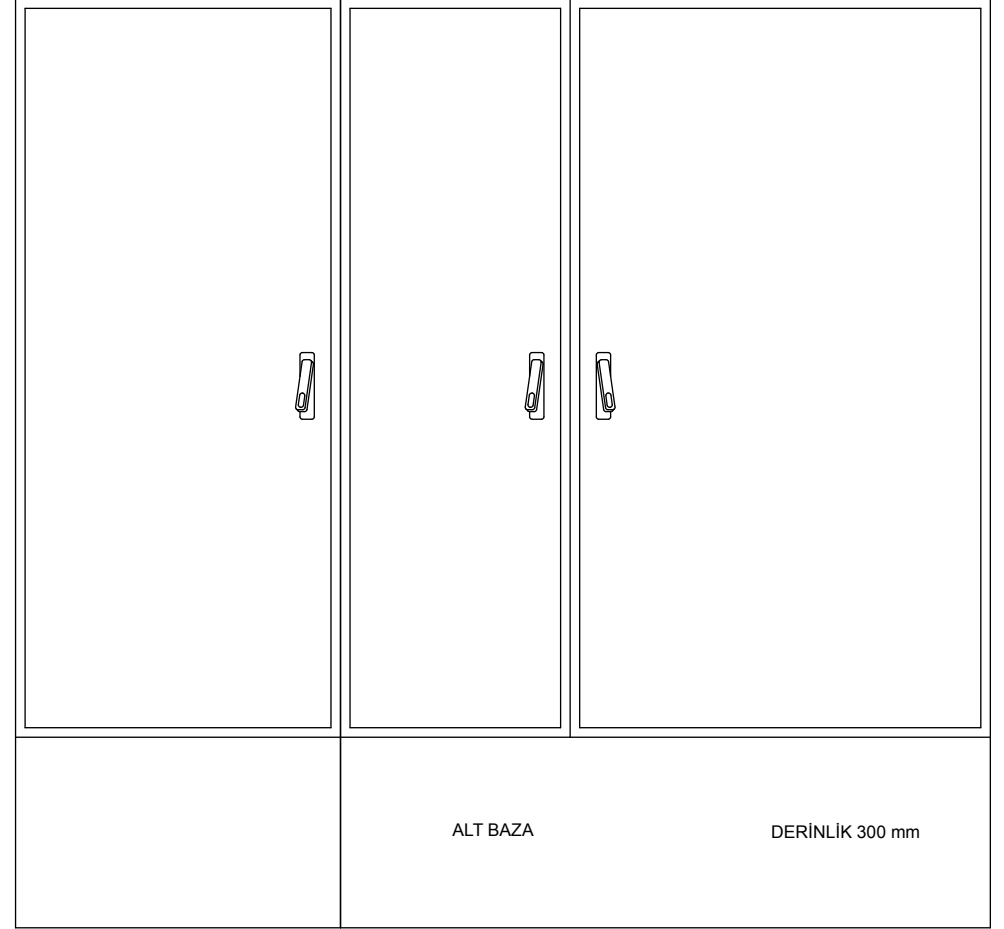
22 TRİFAZE SAYAÇLI DAĞITIM PANOSU
