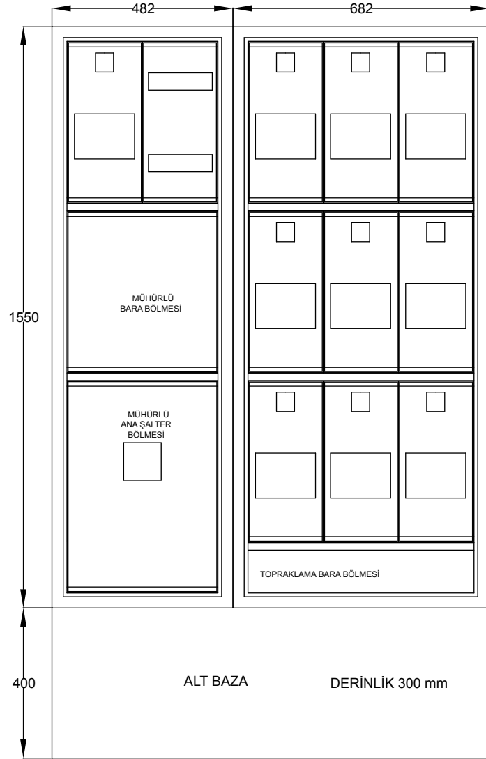
10 TRİFAZE SAYAÇLI DAĞITIM PANOSU
