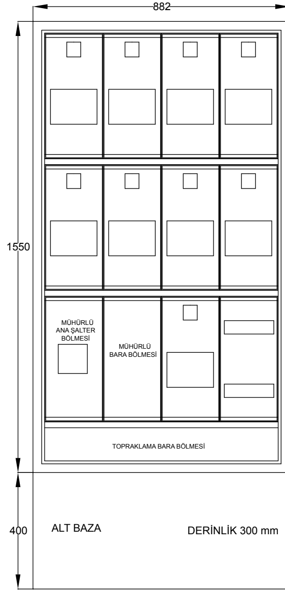
9 TRİFAZE SAYAÇLI DAĞITIM PANOSU
