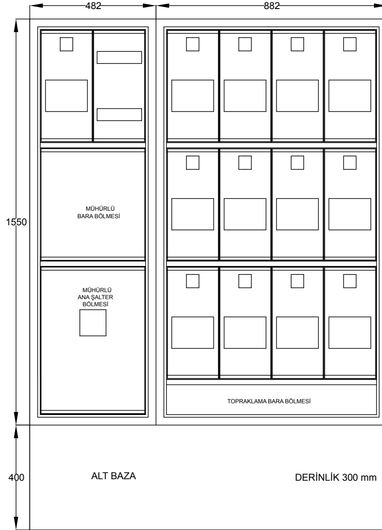
13 TRİFAZE SAYAÇLI DAĞITIM PANOSU
