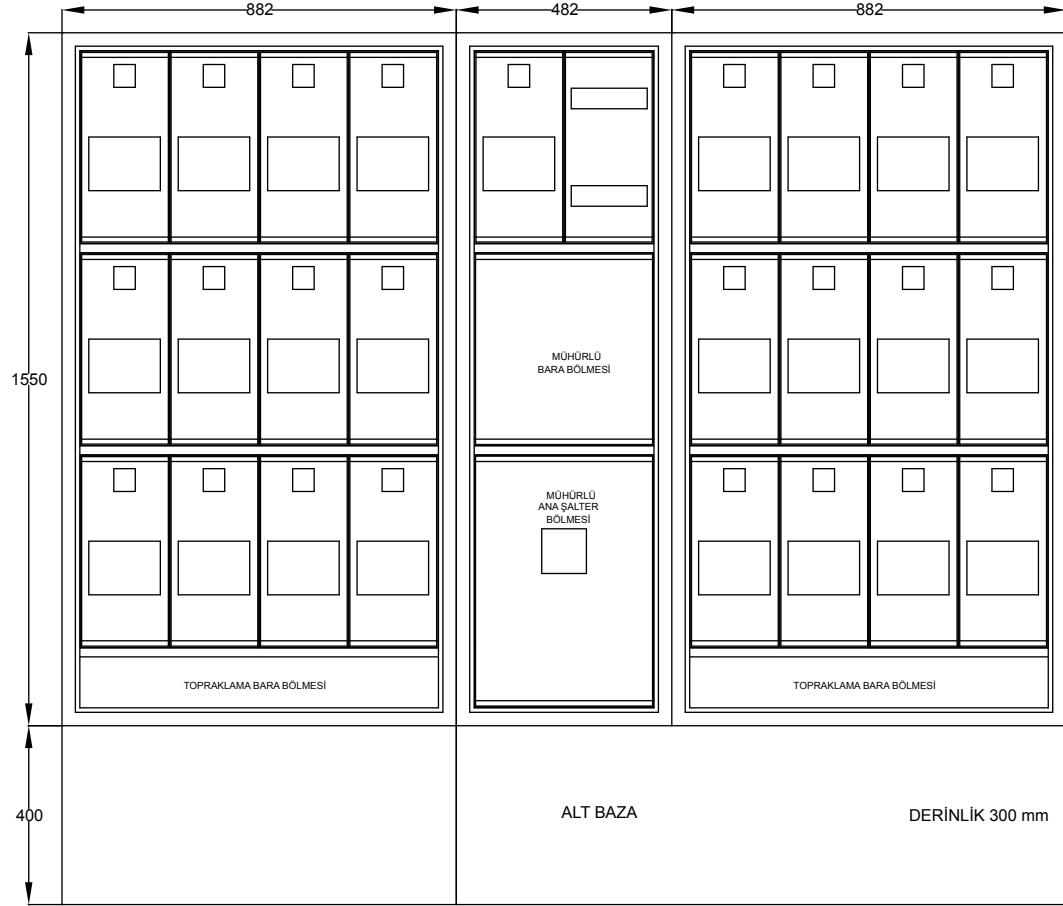
25 TRİFAZE SAYAÇLI DAĞITIM PANOSU
