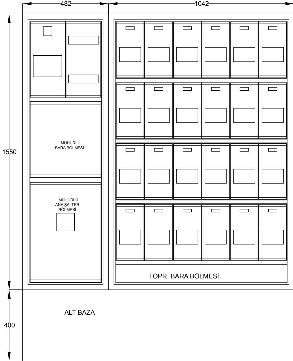
1 TRİFAZE 24 MONOFAZE SAYAÇLI DAĞITIM PANOSU
