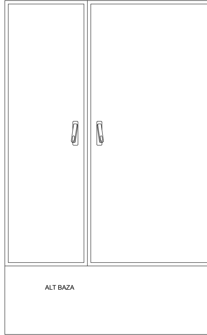
1 TRİFAZE 16 MONOFAZE SAYAÇLI DAĞITIM PANOSU DIŞ GÖRÜNÜŞÜ
