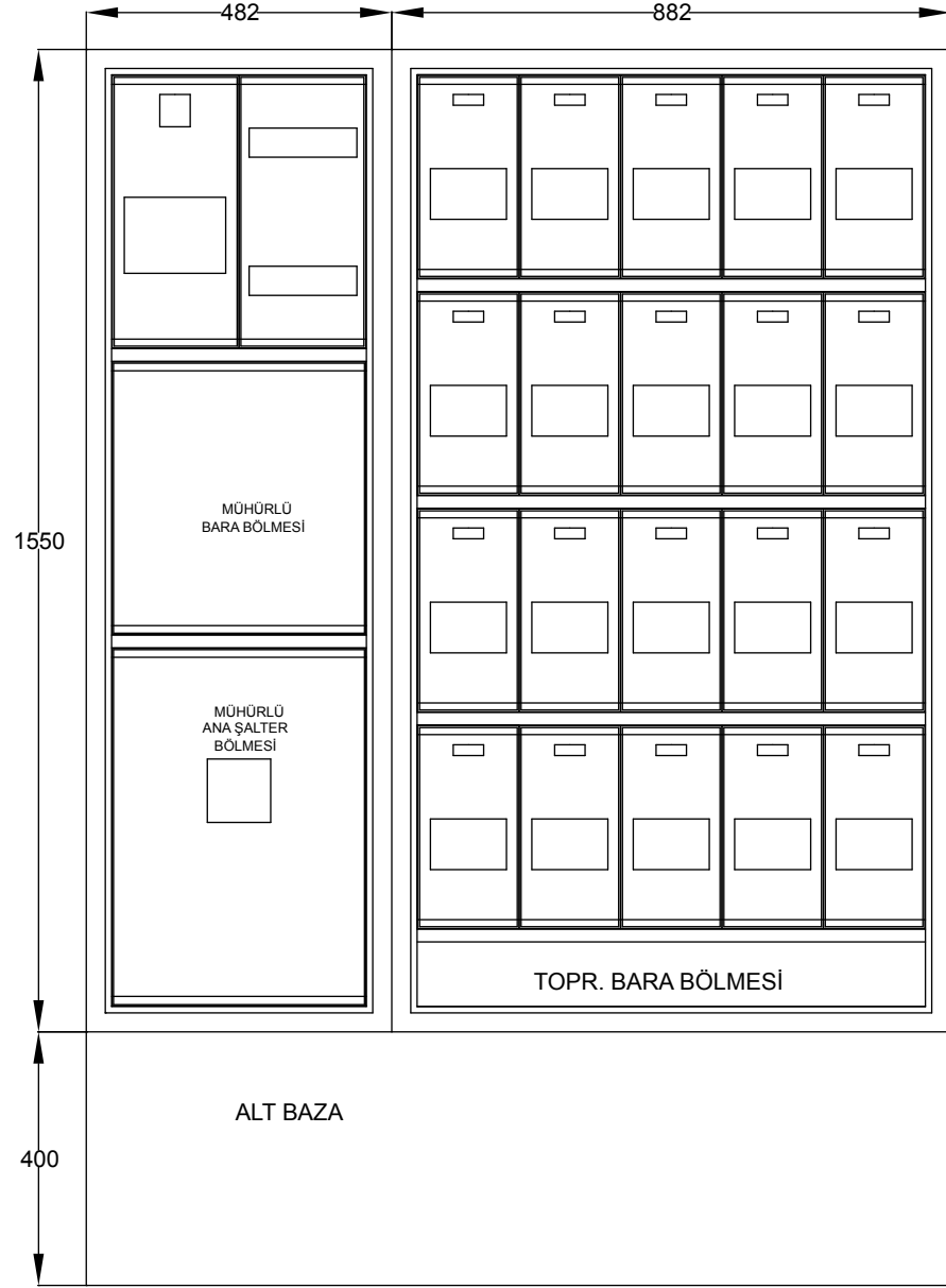
1 TRİFAZE 20 MONOFAZE SAYAÇLI DAĞITIM PANOSU
