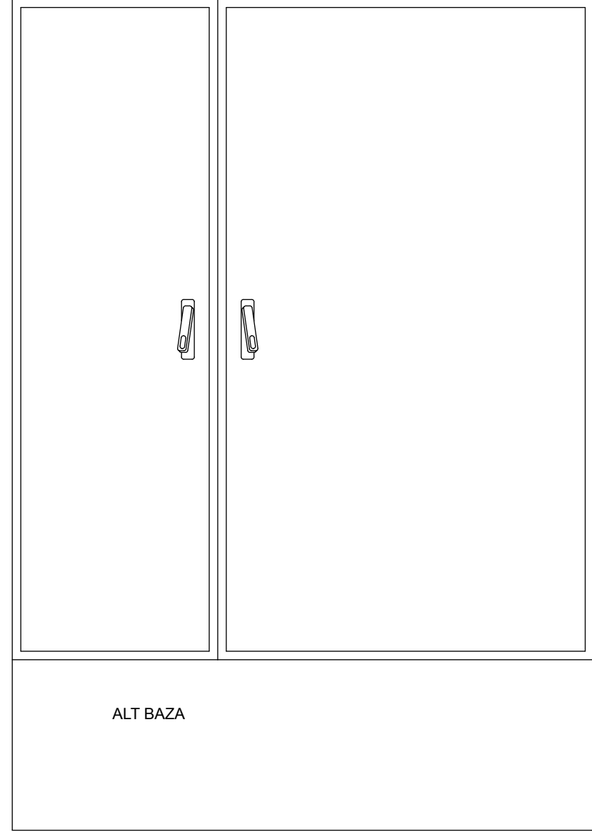
1 TRİFAZE 20 MONOFAZE SAYAÇLI DAĞITIM PANOSU DIŞ GÖRÜNÜŞ
