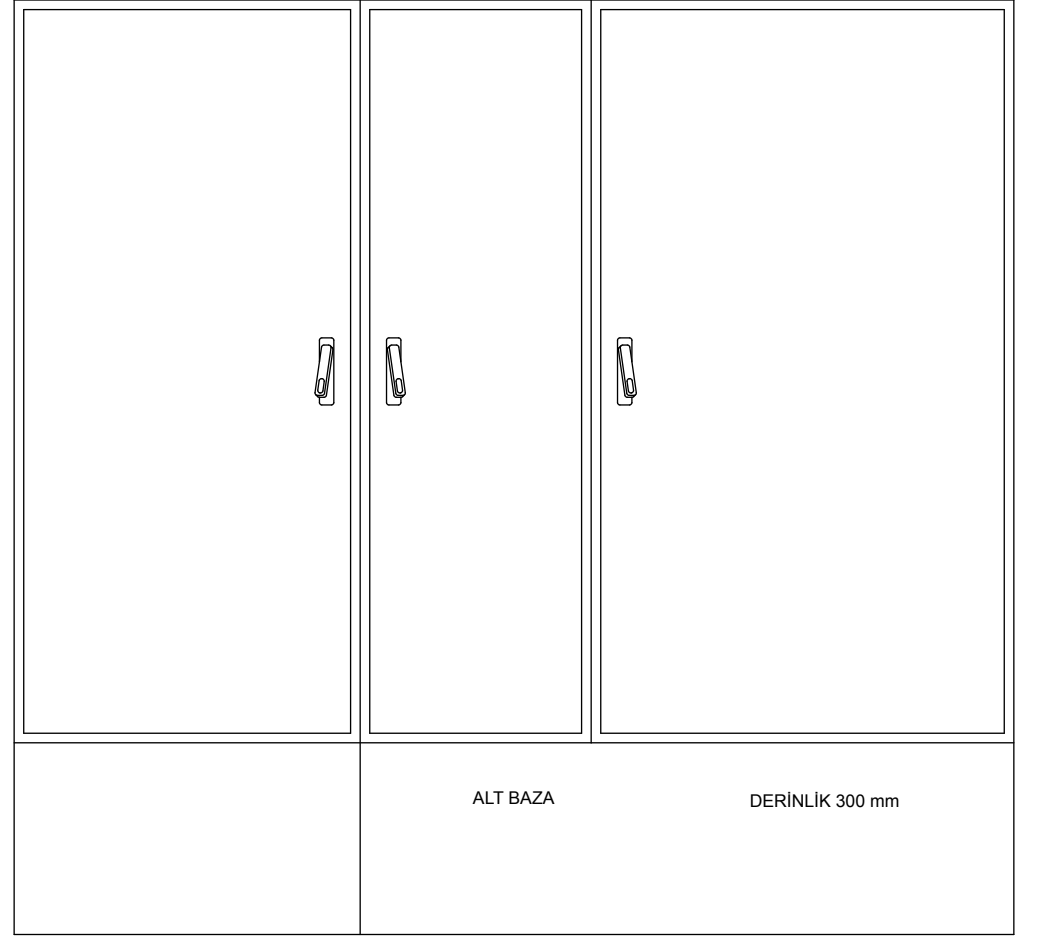
1 TRİFAZE 36 MONOFAZE SAYAÇLI DAĞITIM PANOSU
