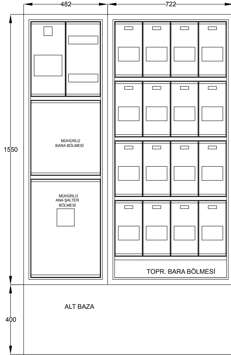
1 TRİFAZE 16 MONOFAZE SAYAÇLI DAĞITIM PANOSU
