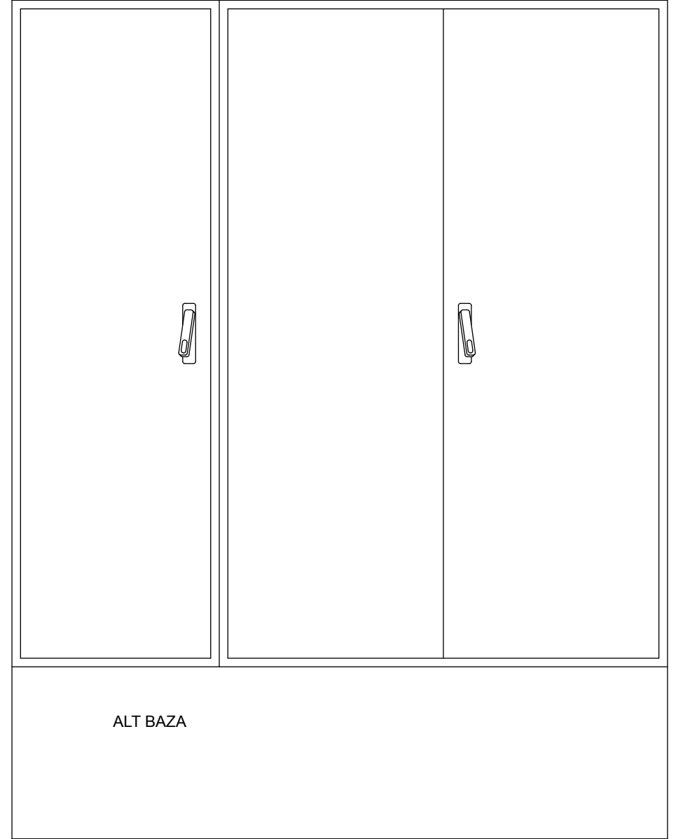
1 TRİFAZE 24 MONOFAZE SAYAÇLI DAĞITIM PANOSU DIŞ GÖRÜNÜŞ
