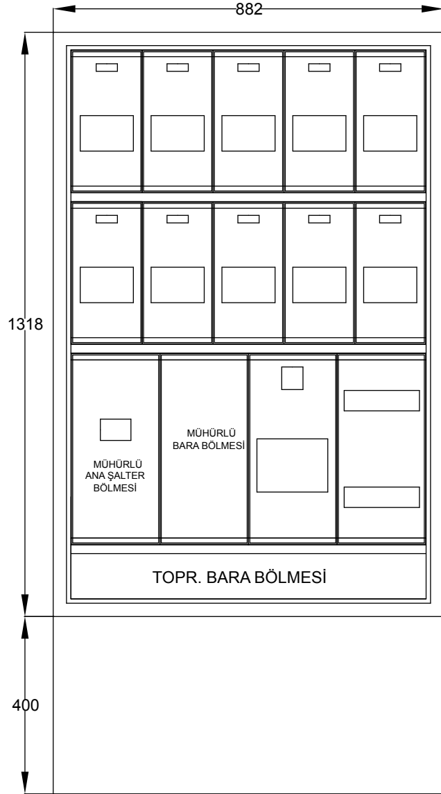
1 TRİFAZE 10 MONOFAZE SAYAÇLI DAĞITIM PANOSU
